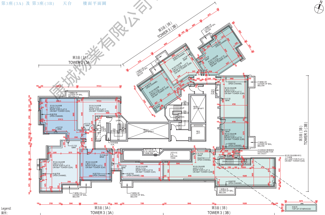
Tower 3(3A) & Tower 3(3B) Roof Floor Plan 第3座(3A)及第3座(3B) 天台 樓面平面圖
